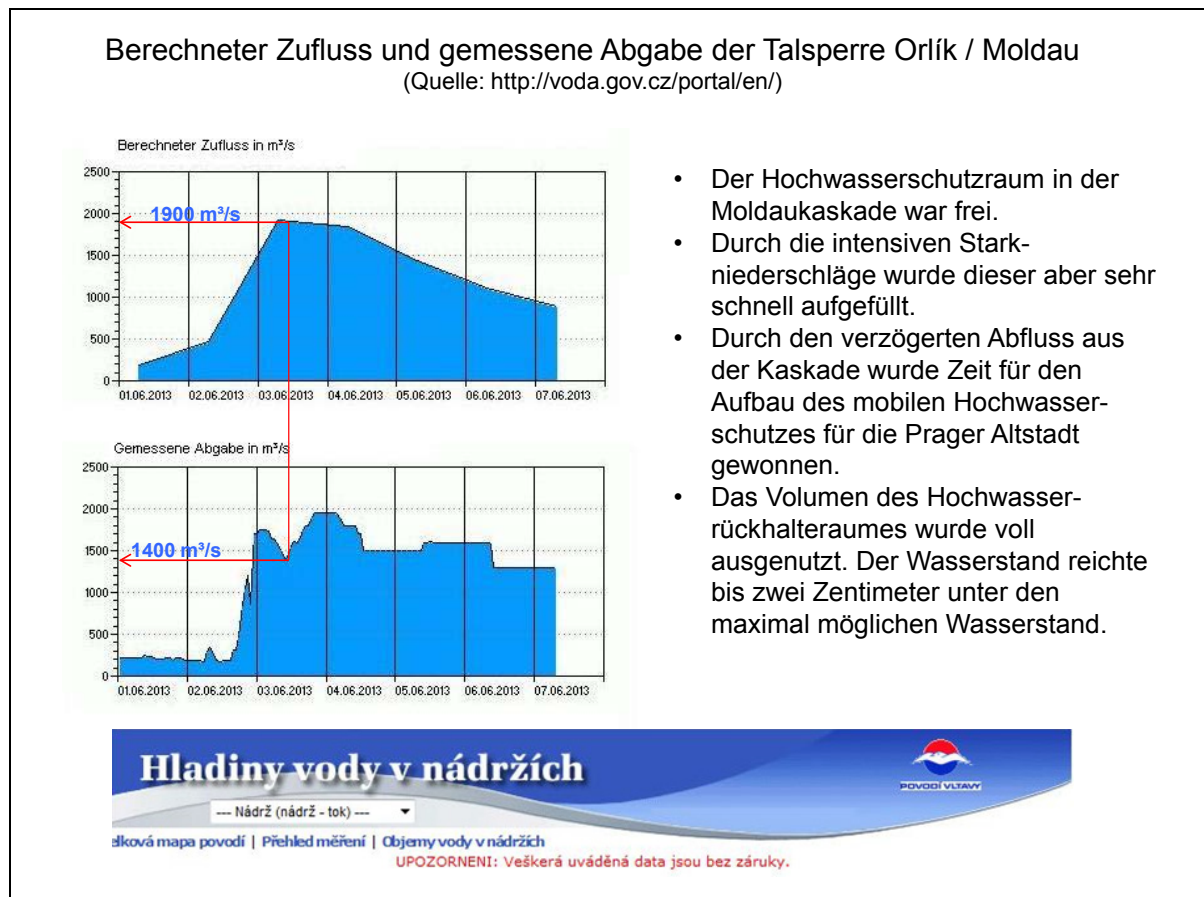
Abb. 12: Wasserrückhalt der Talsperre Orlík, Moldau (Quelle: POVODI Vltava, LfULG) 25
